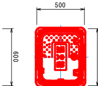
φ75用(土盛り1000)
