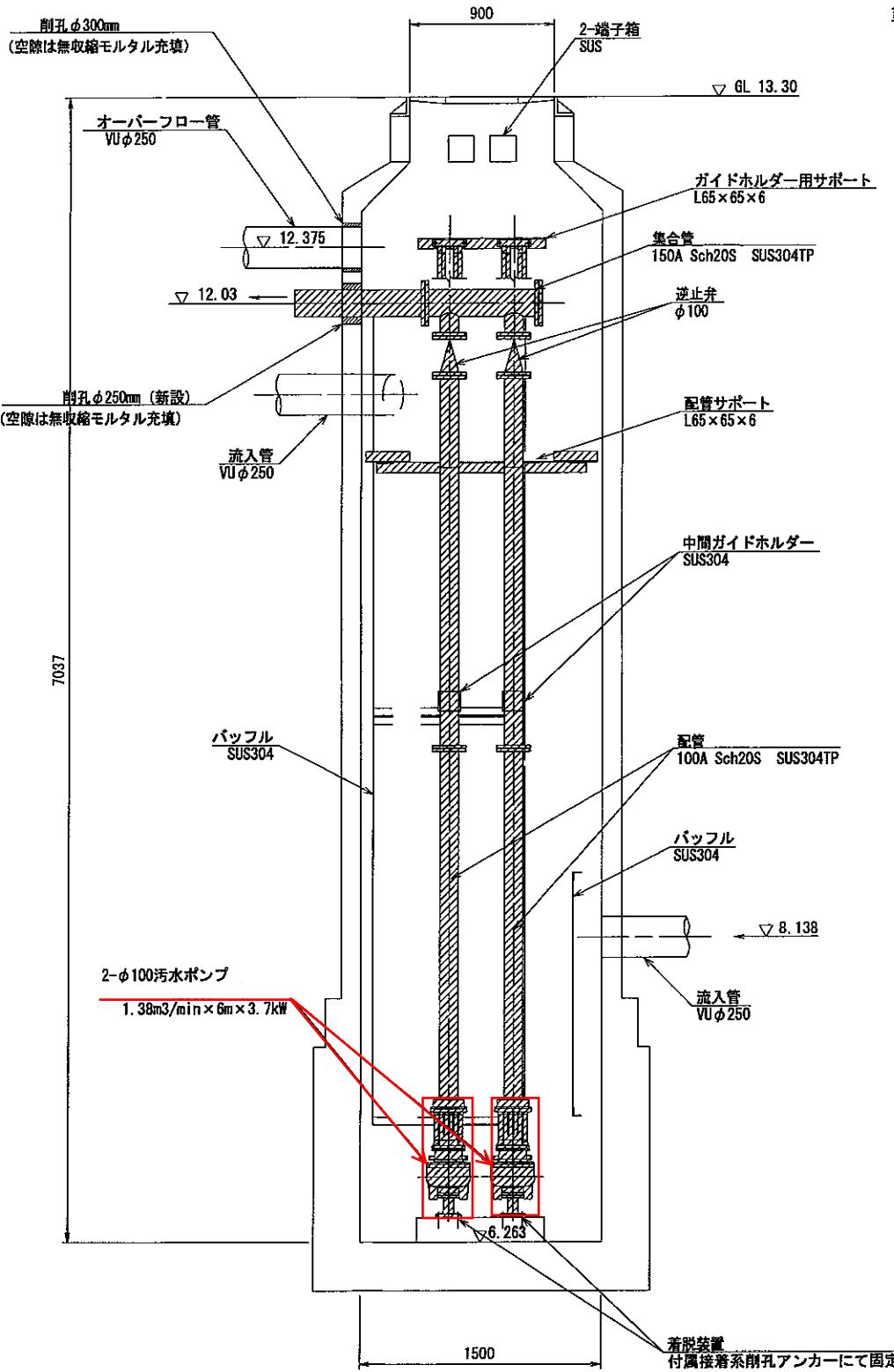
B-B断面図
