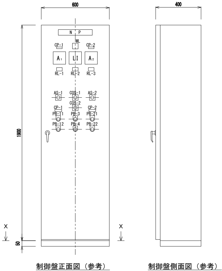
制御盤正面図（参考）
