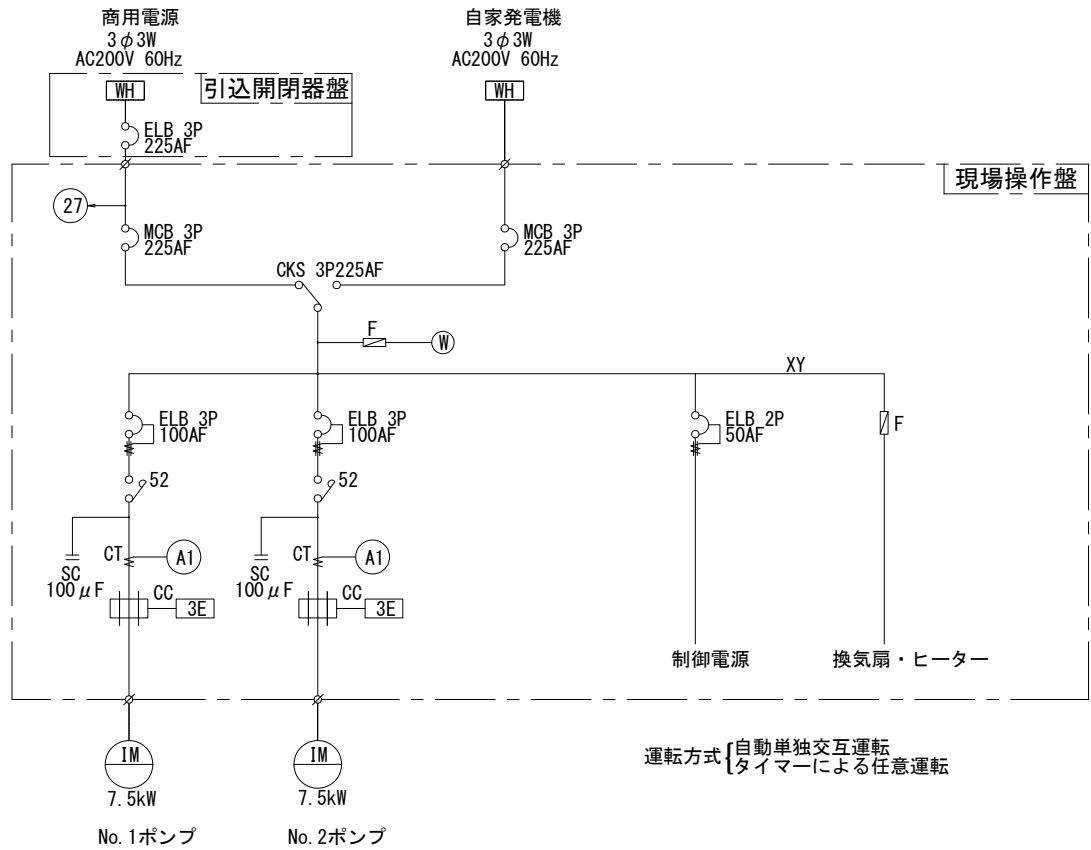
単線結線図（参考）
