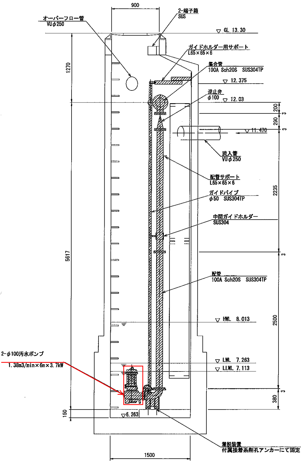
A-A断面図
