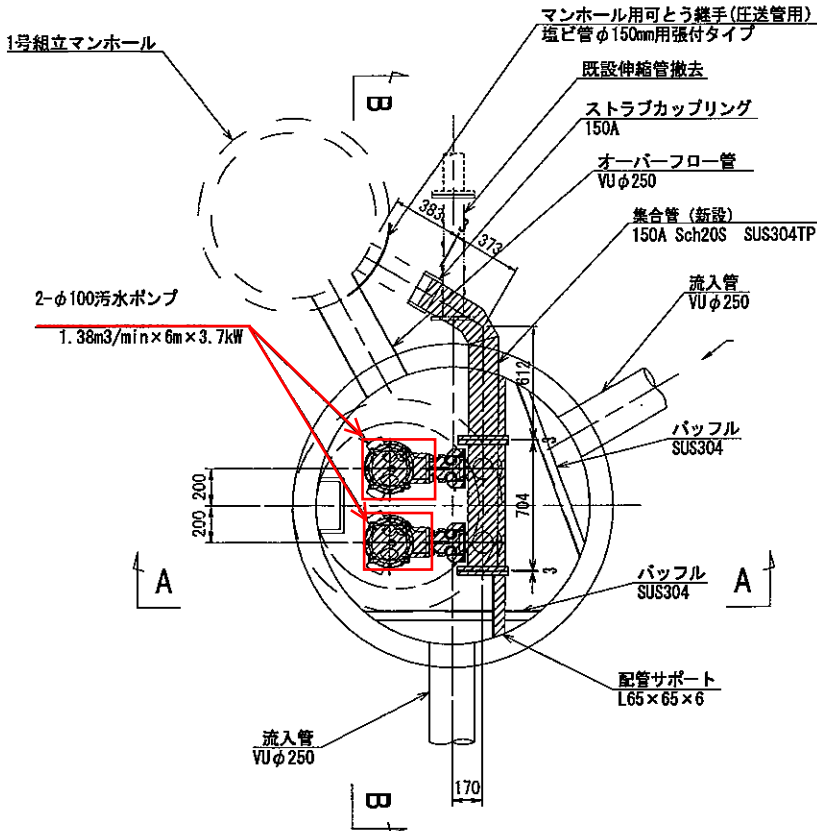
平面図
