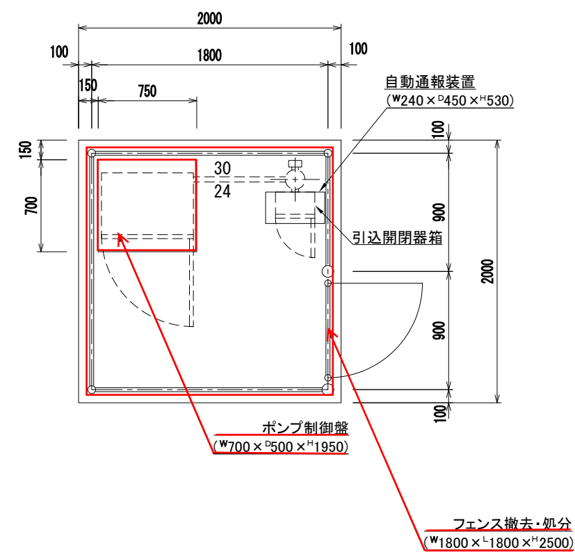
機器配置図 S=1/20
