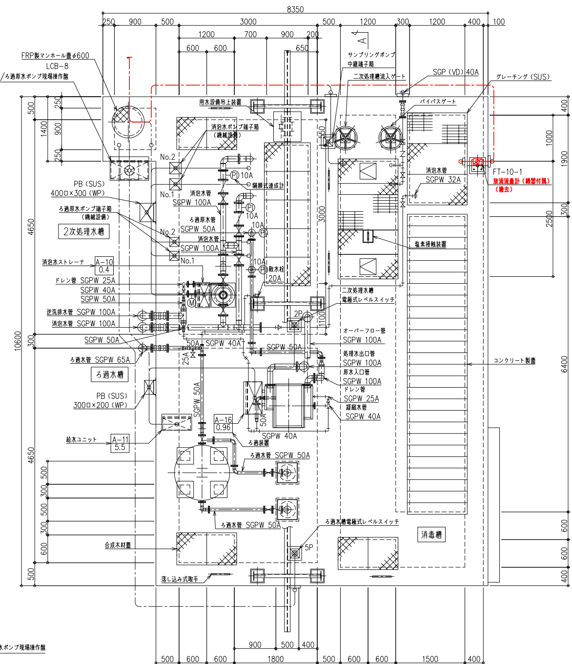
1F平面図
