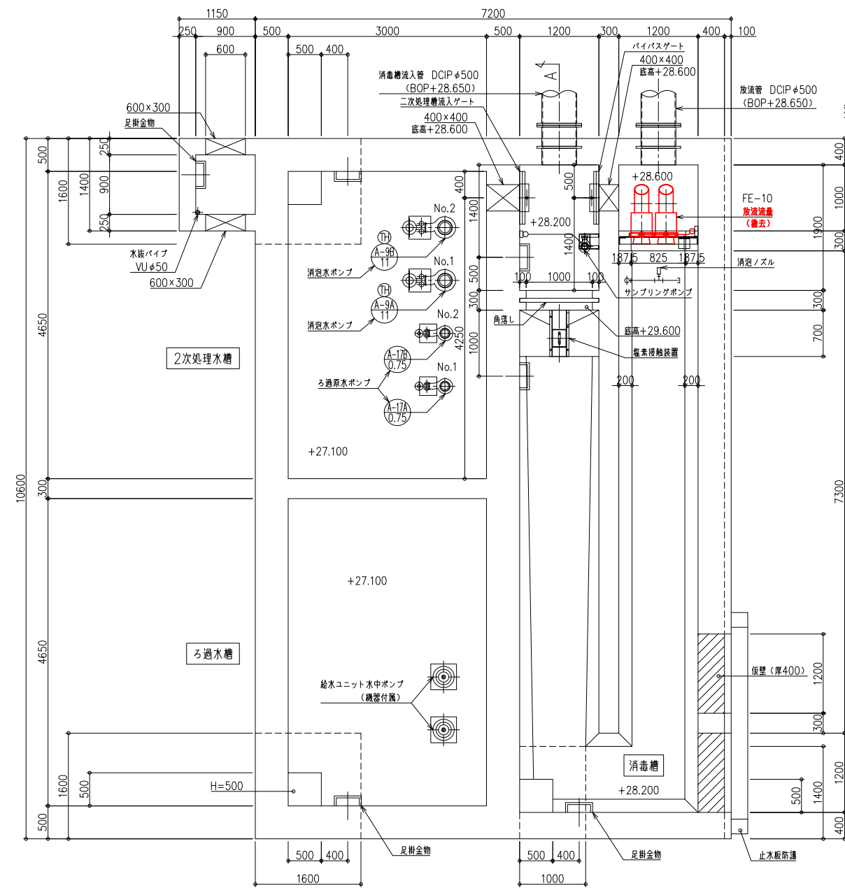
B1F平面図
