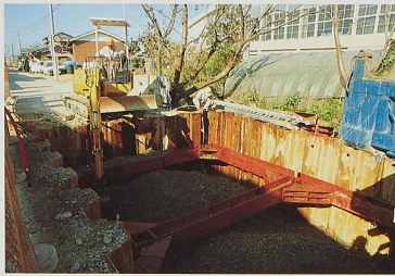
▲上水道配水施設
