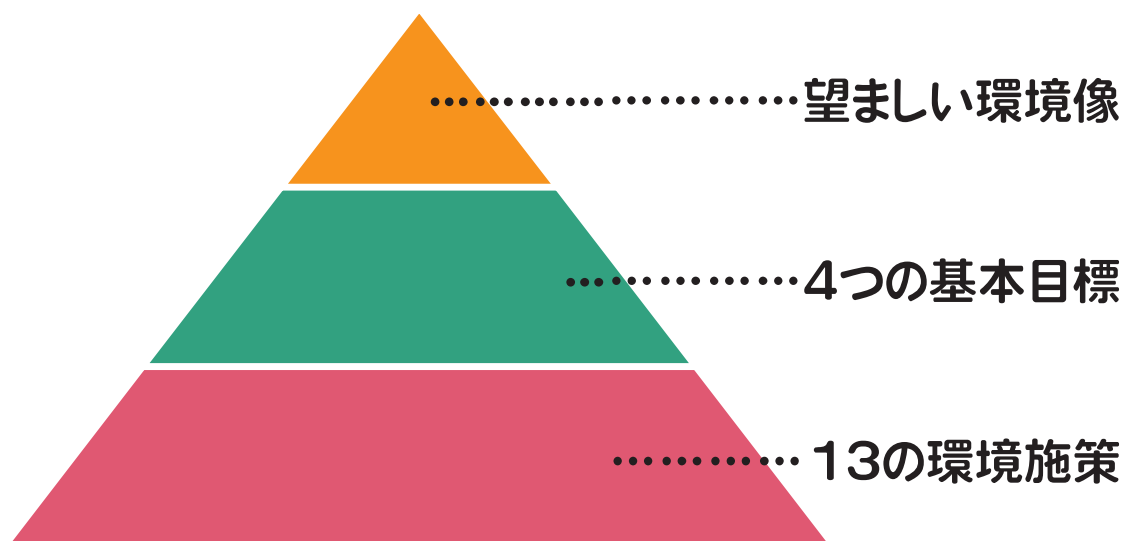
図3-1 施策体系図
