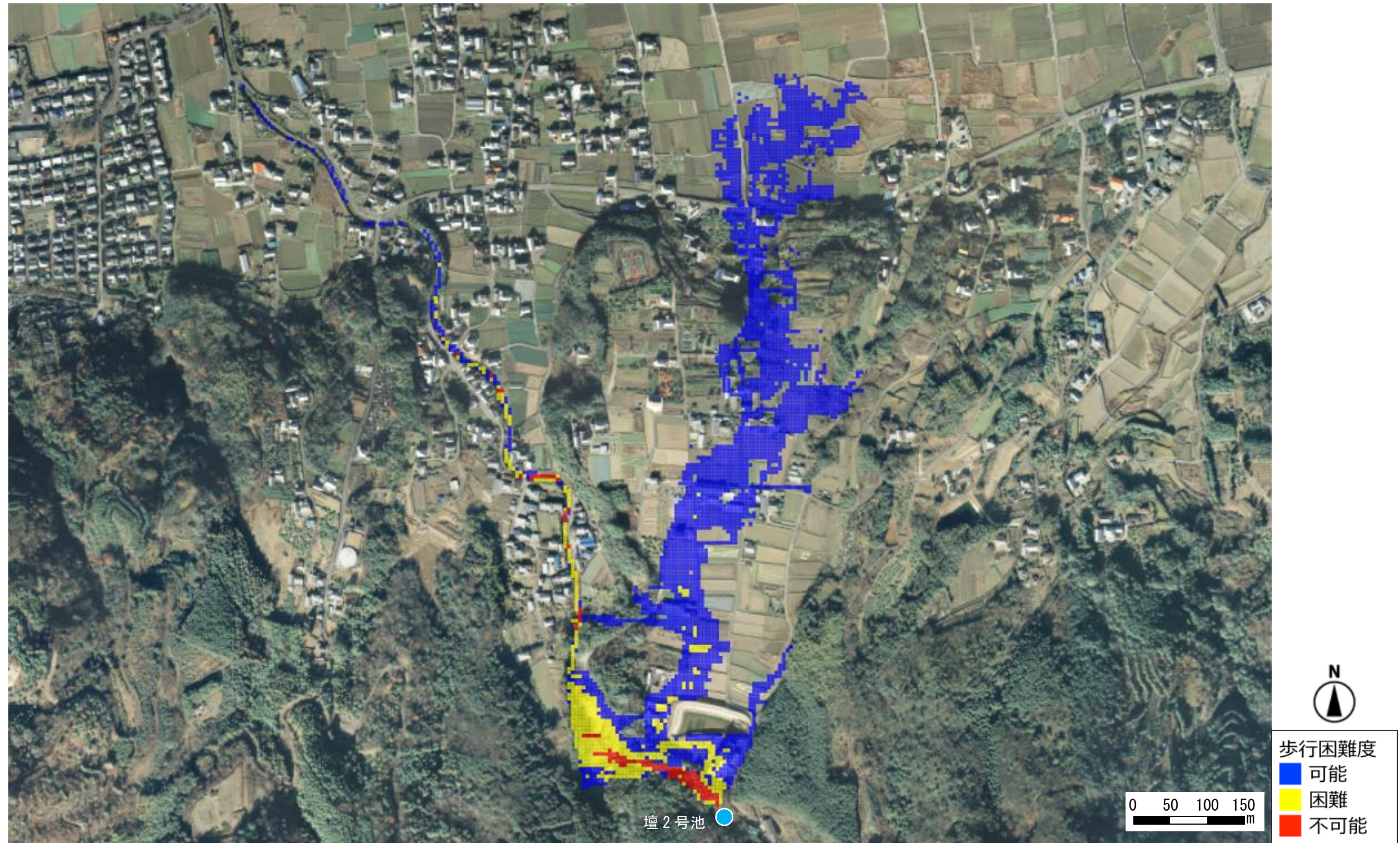
壇 2 号池浸水想定区域図（最大歩行困難度）
