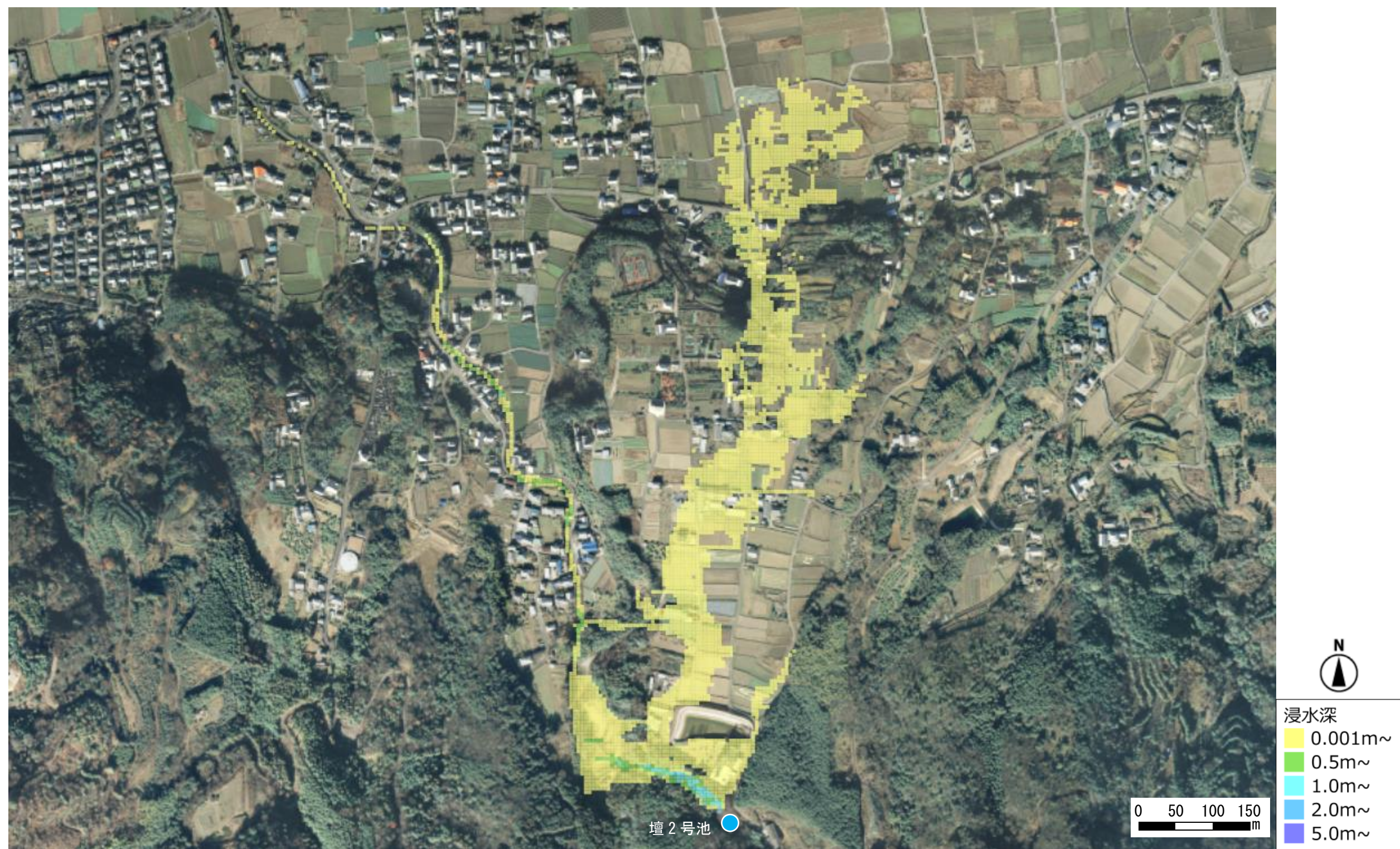
壇 2 号池浸水想定区域図（最大浸水深）
