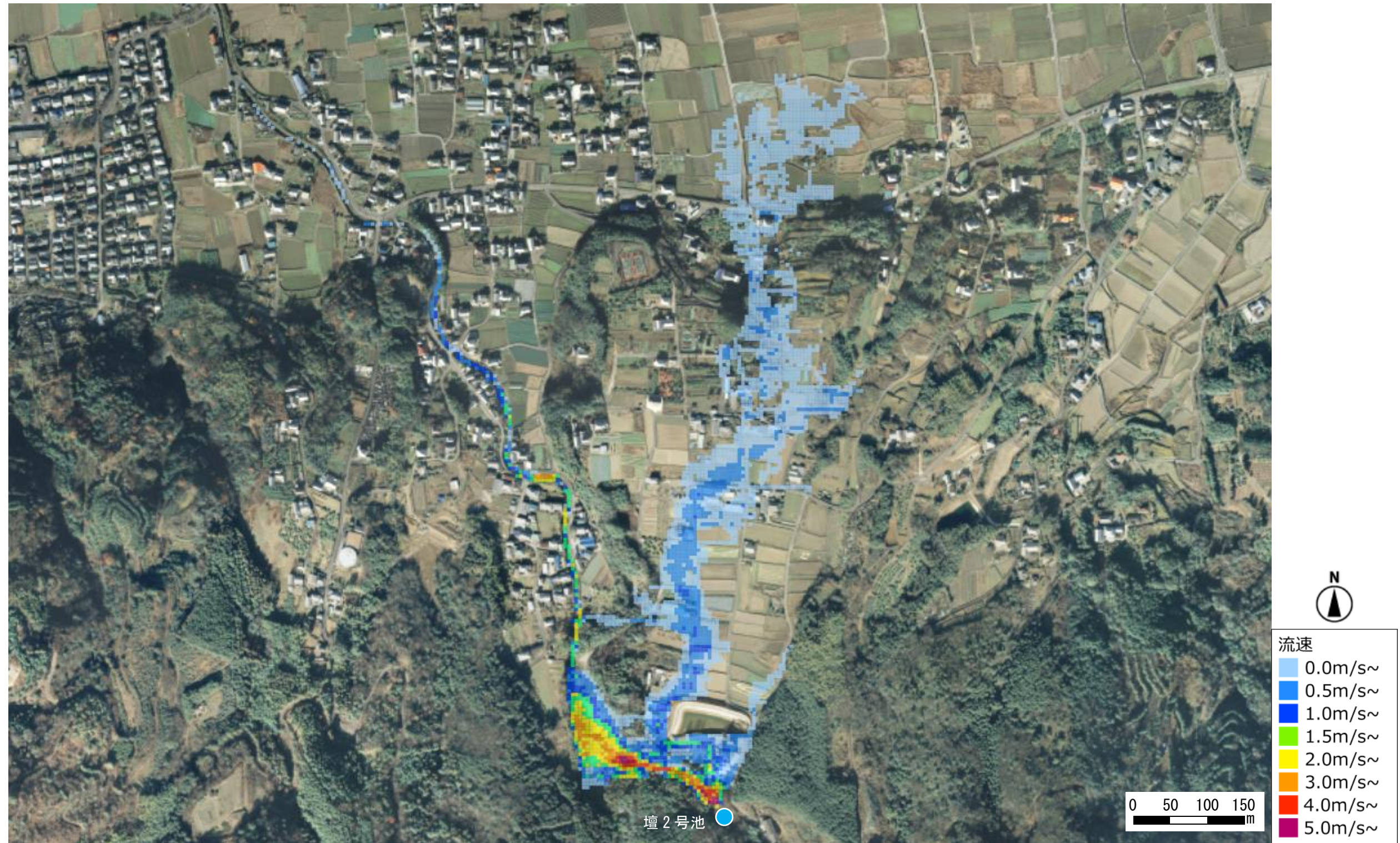
壇 2 号池浸水想定区域図（最大流速）
