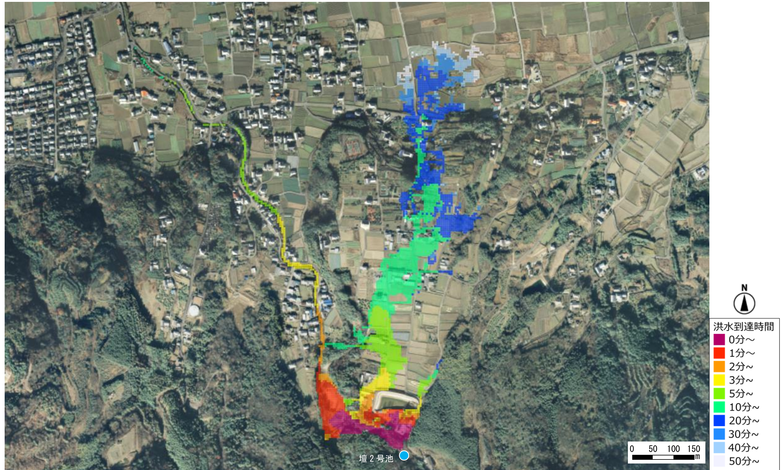
壇 2 号池浸水想定区域図（洪水到達時間）
