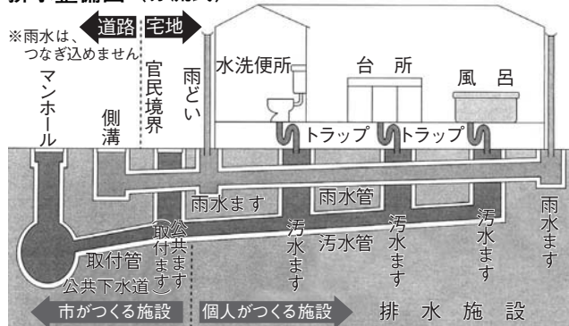
排水整備図（分流式）
